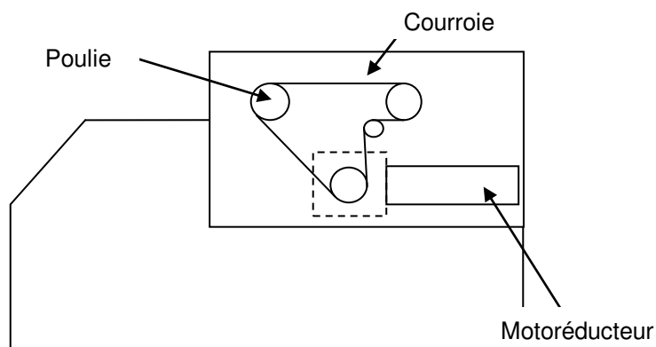
Entrainement bobine
