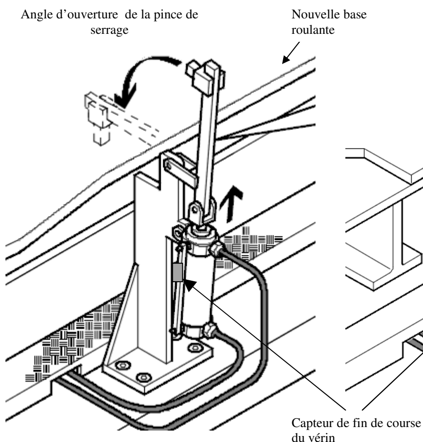
PINCE EN POSITION OUVERTE
